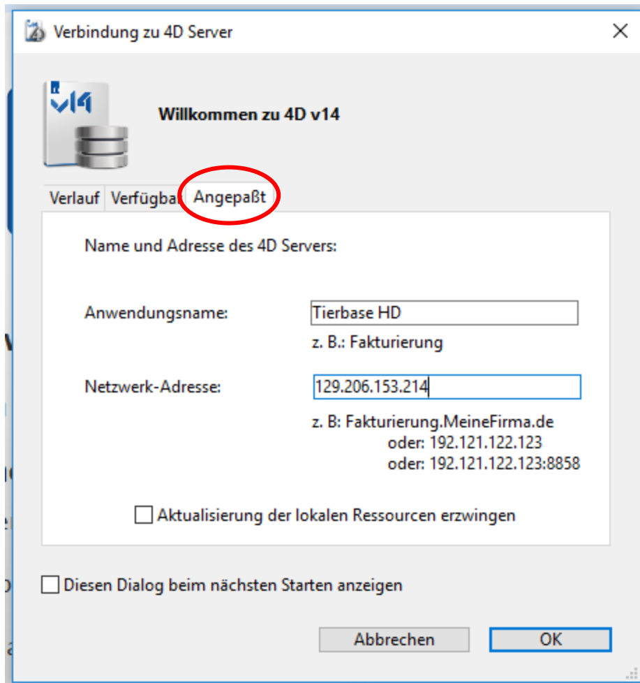
Abb. 3: Server Anmeldung, Maske für notwendige Eingaben, roter Kreis markiert korrekte Eingabemaske.
